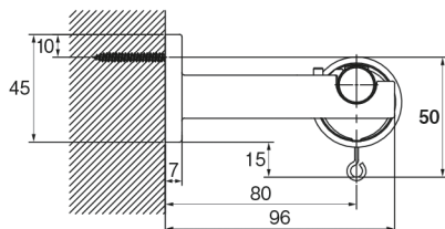
シングルブラケット付（ブラケット幅=20mm）
