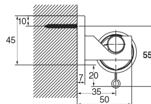
天井付シングルブラケット付（ブラケット幅=20mm）
