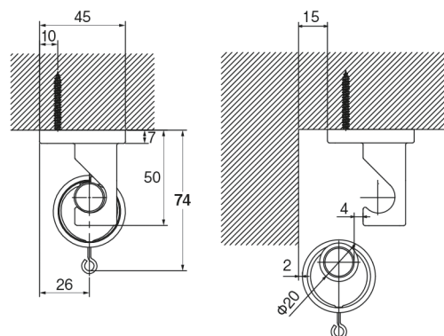
天井付シングルブラケット付（ブラケット幅=20mm）
